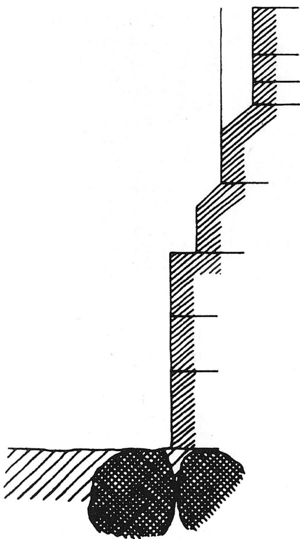
Fig. 6. Profil af soklen på Sct. Budolfi kirkes apsis (Tegning Torben Hjelm).
