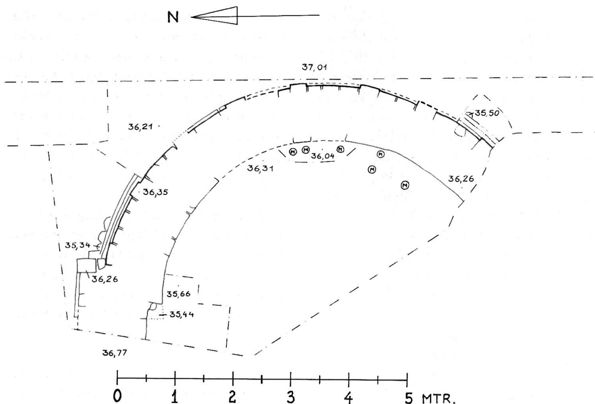
Fig. 4. Den udgravede del af apsis og kor. Plan fra undersøgelsen 1981 (Tegning Torben Hjelm).
